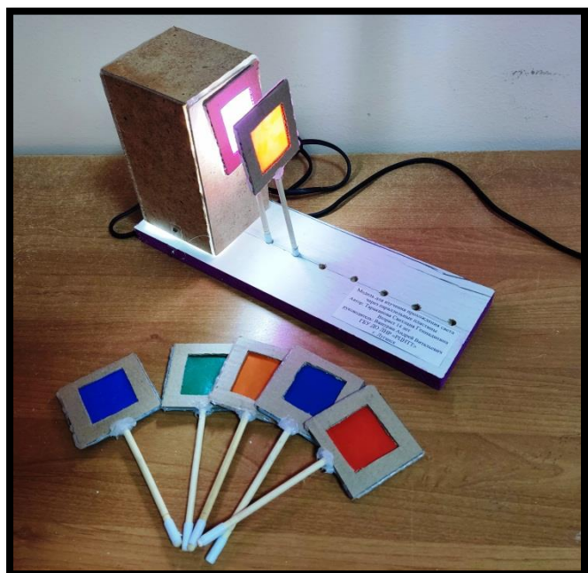
«Модель для изучения прохождения света через параллельные пластины» Тараканова Светлана, секция «Физика» НО «РМАН» ГБУ ДО ЛНР «Республиканский центр научно - технического творчества» (пед. доп. обр. Вашурин А.В.)
